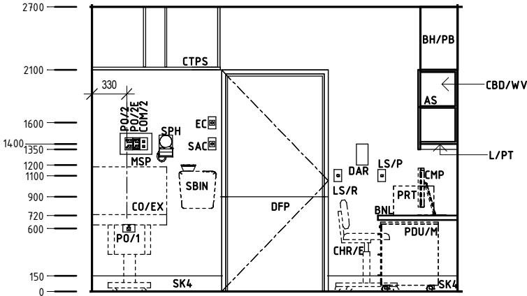
Elevation 3
