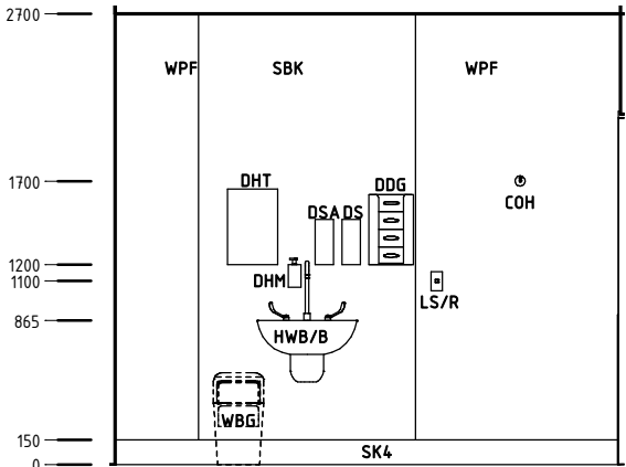
Elevation 2
