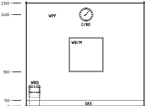
Elevation 1
