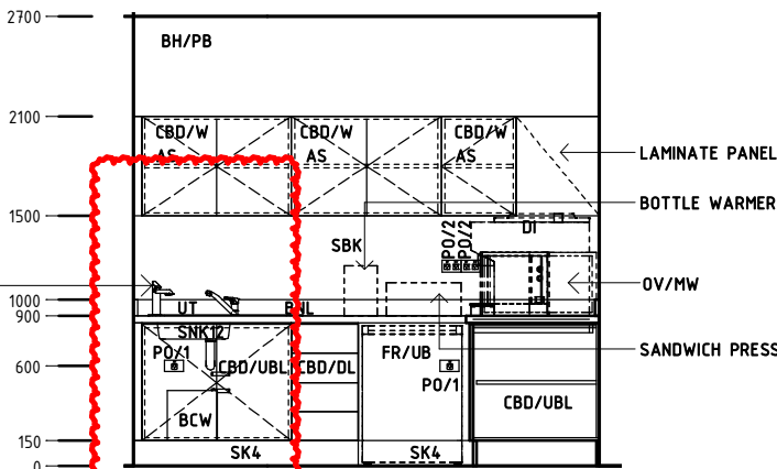
Elevation 4
