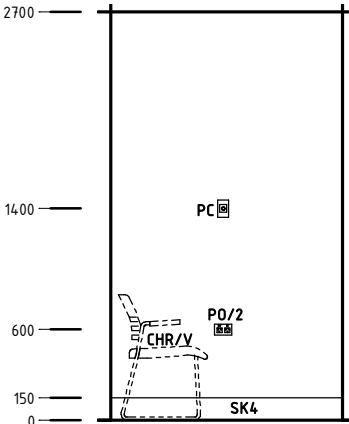
Elevation 1
