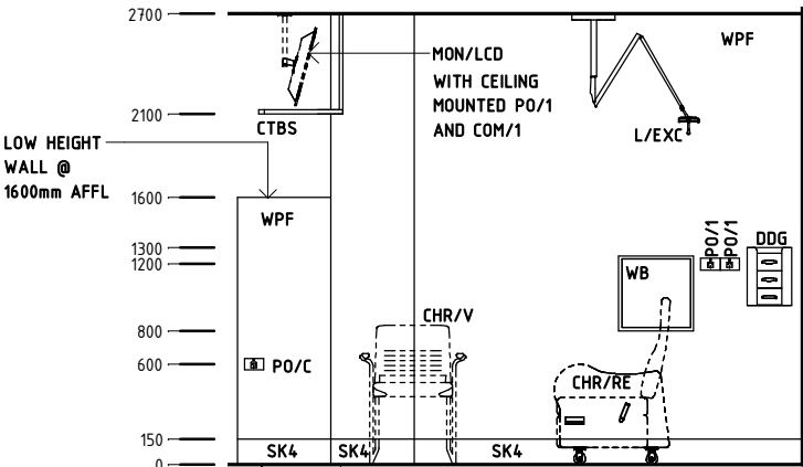
Elevation 4
