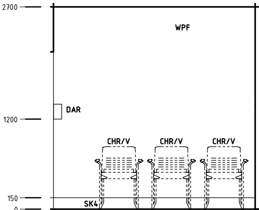
Elevation 4
