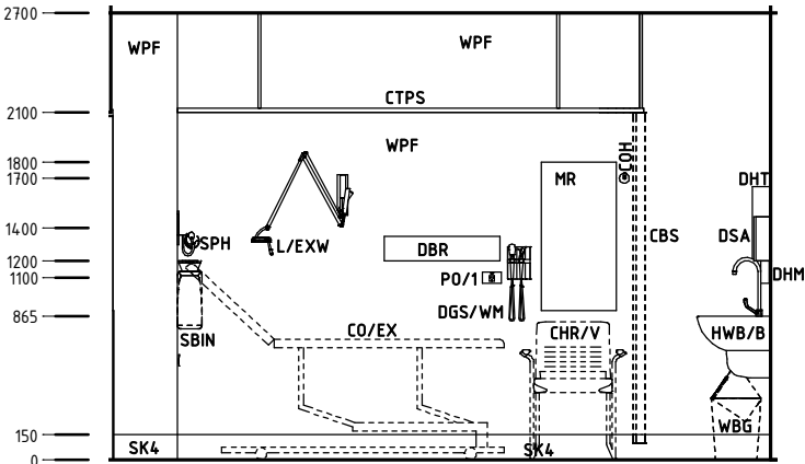
Elevation 1
