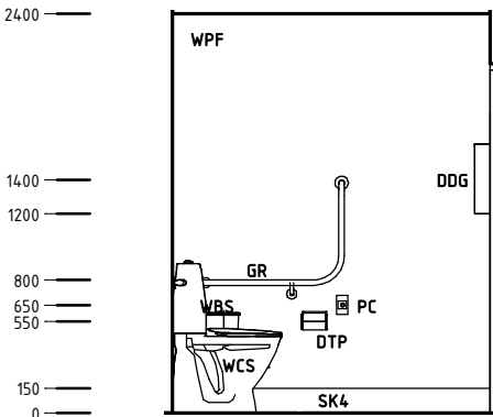
Elevation 2
