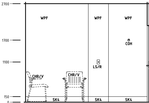
Elevation 4
