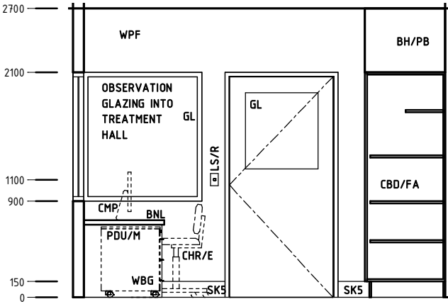
Elevation 2
