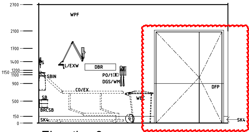
Elevation 3
