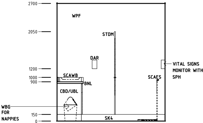
Elevation 4
