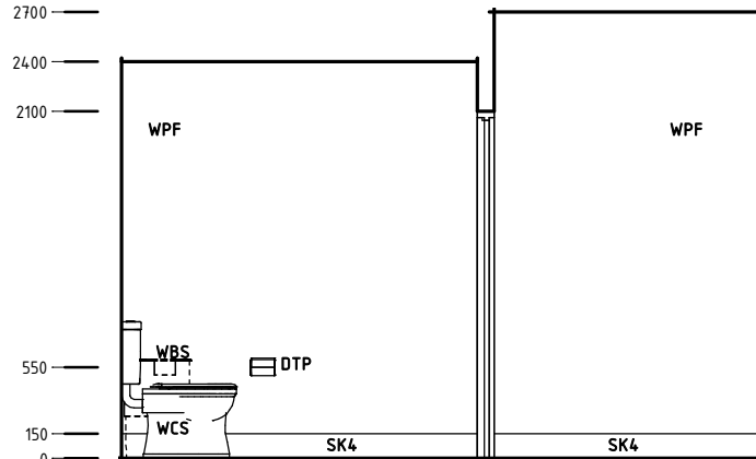
Elevation 4
