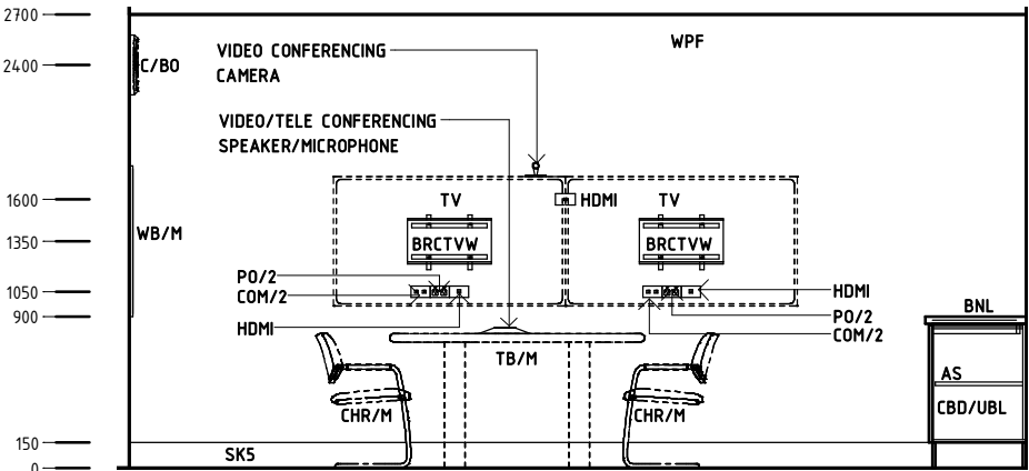
Elevation 3
