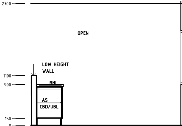
Elevation 3
