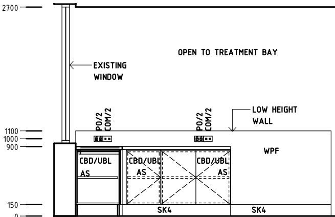
Elevation 2
