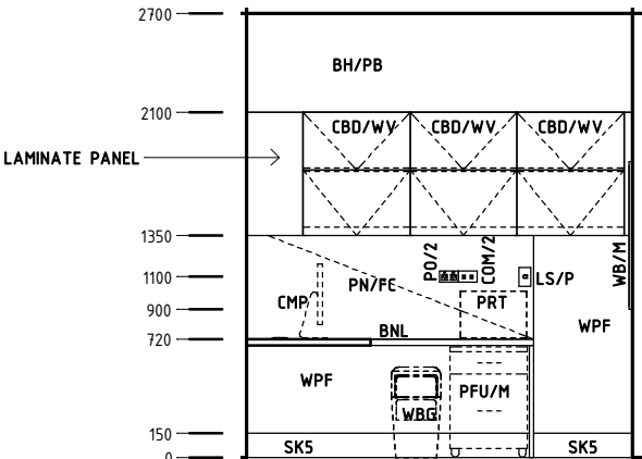
Elevation 2
