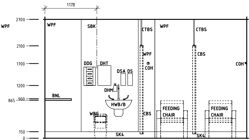
Elevation 3
