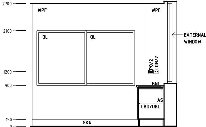
Elevation 4
