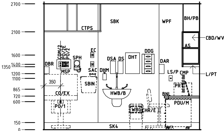
Elevation 2
