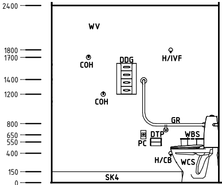
Elevation 1
