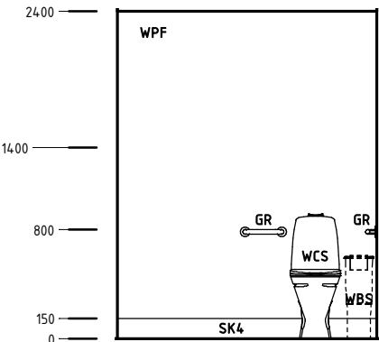
Elevation 1
