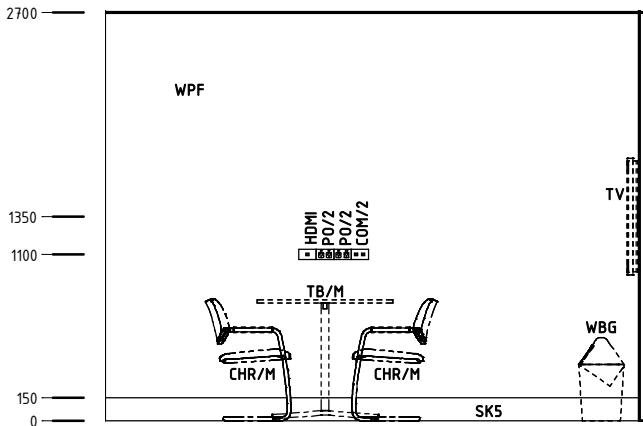
Elevation 3
