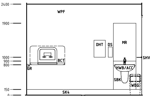
Elevation 2
