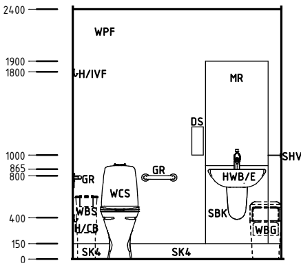
Elevation 1
