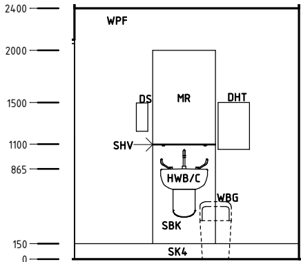
Elevation 6
