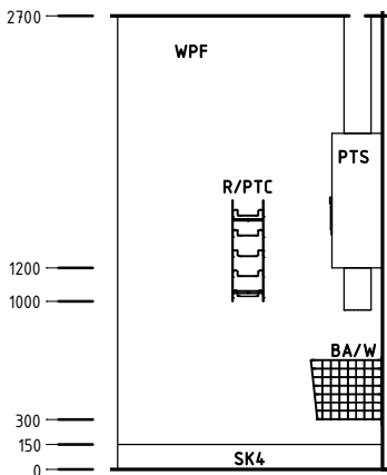
Elevation 1
