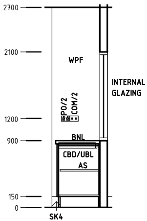
Elevation 4
