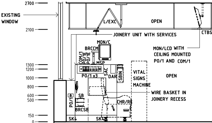
Elevation 2
