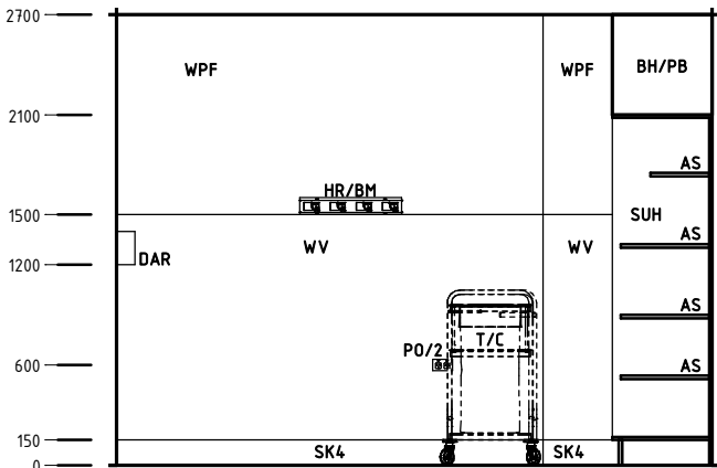
Elevation 4
