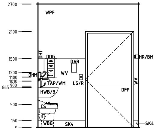
Elevation 3
