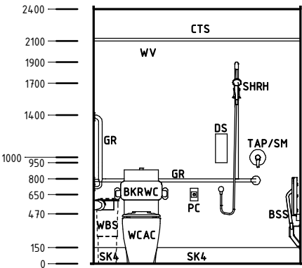
Elevation 1
