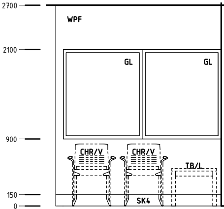
Elevation 3
