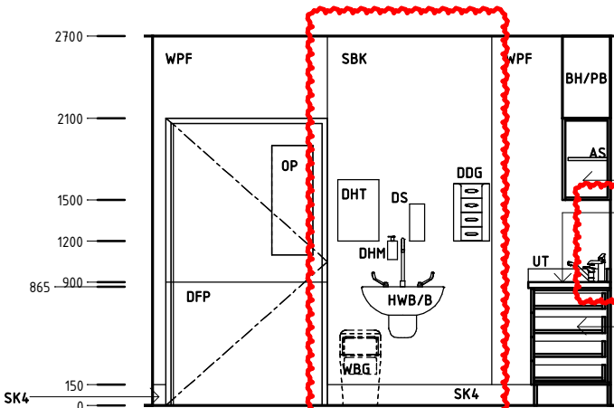
Elevation 3
