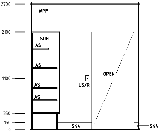
Elevation 2
