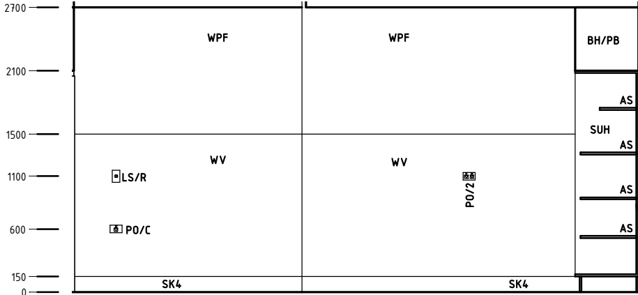
Elevation 3
