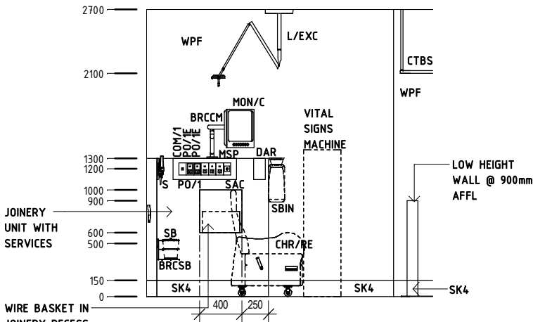
Elevation 5
