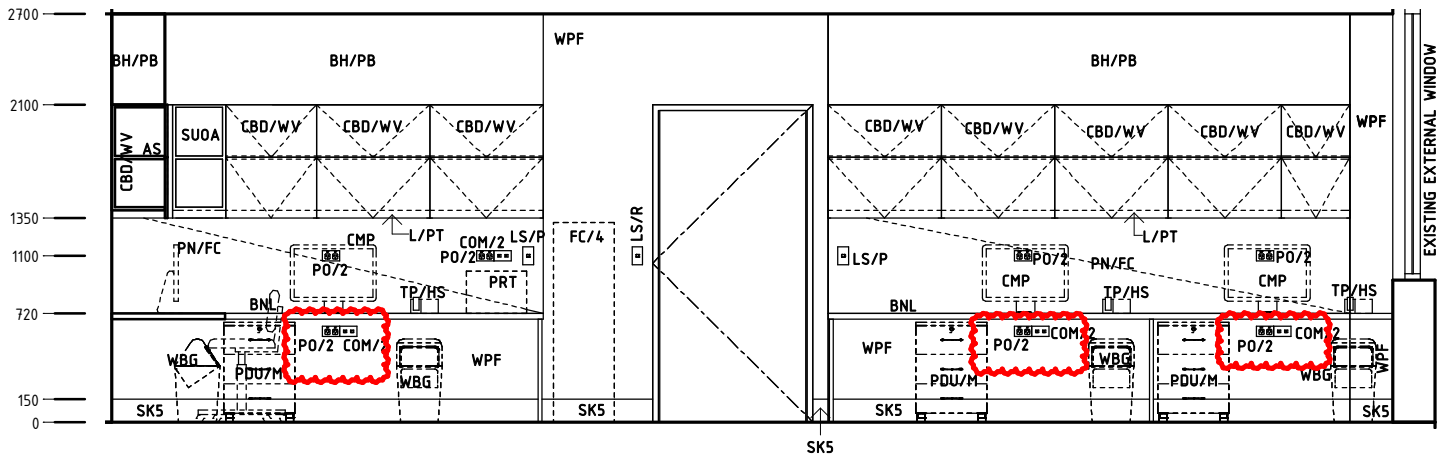
Elevation 4
