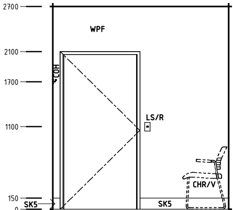
Elevation 4
