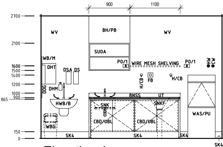
Elevation 4
