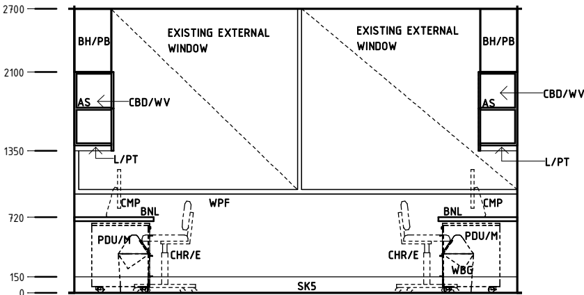
Elevation 1
