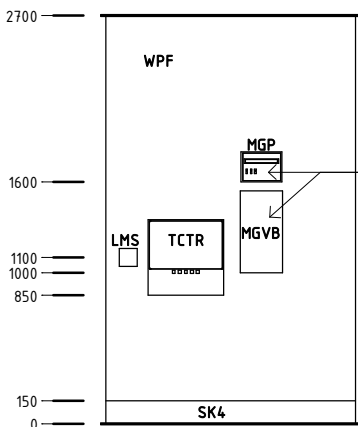
Elevation 10
