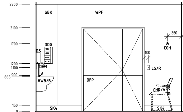
Elevation 3
