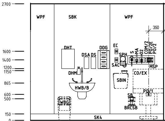
Elevation 2
