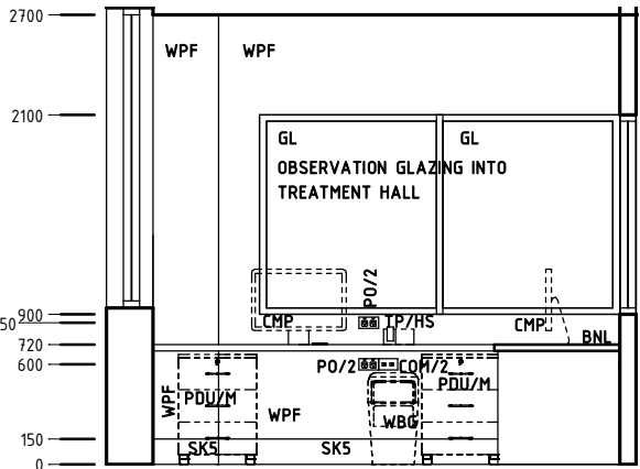
Elevation 2
