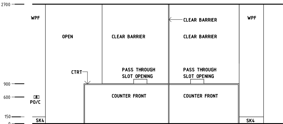
Elevation 6
