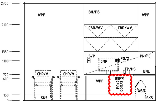
Elevation 4
