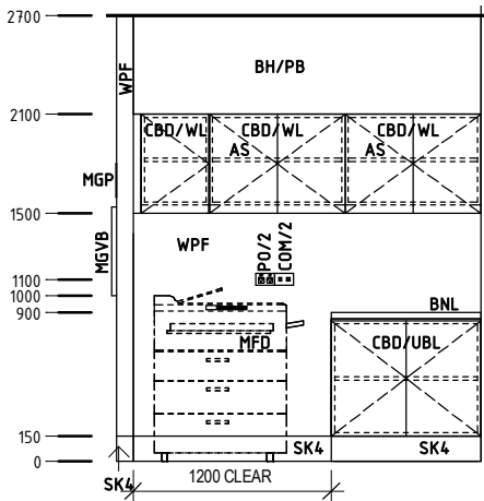
Elevation 7
