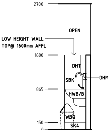
Elevation 1
