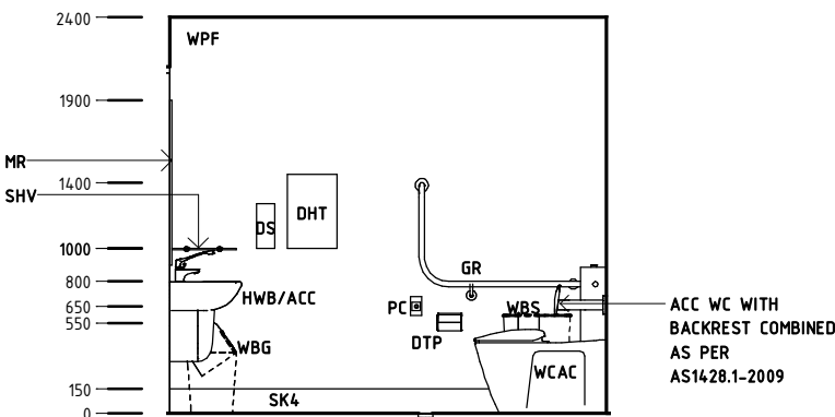
Elevation 4
