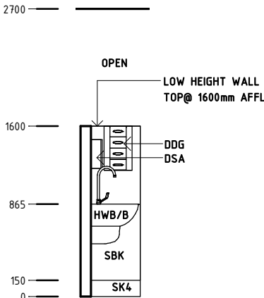
Elevation 3
