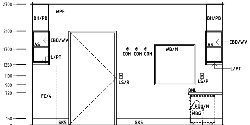
Elevation 3
