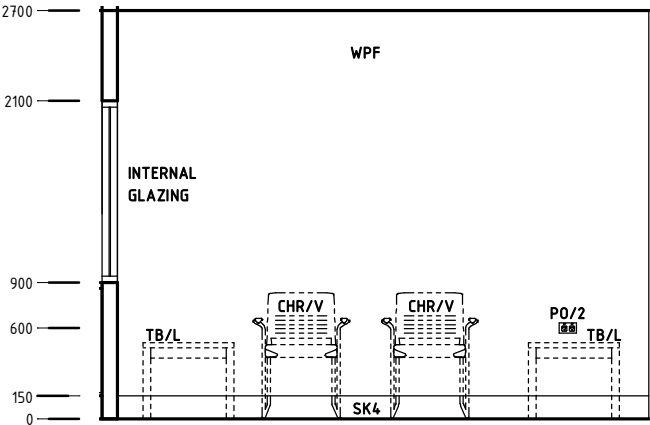
Elevation 1
