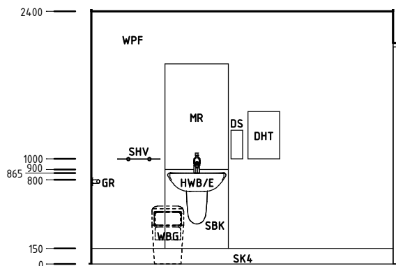
Elevation 4
