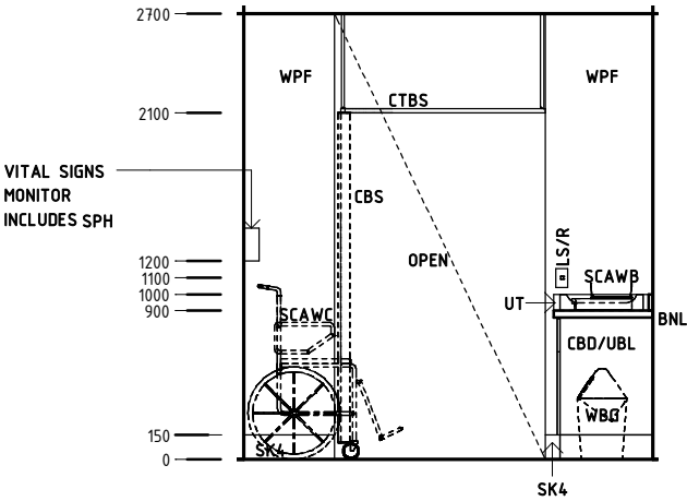
Elevation 2
