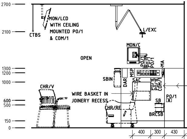
Elevation 5
