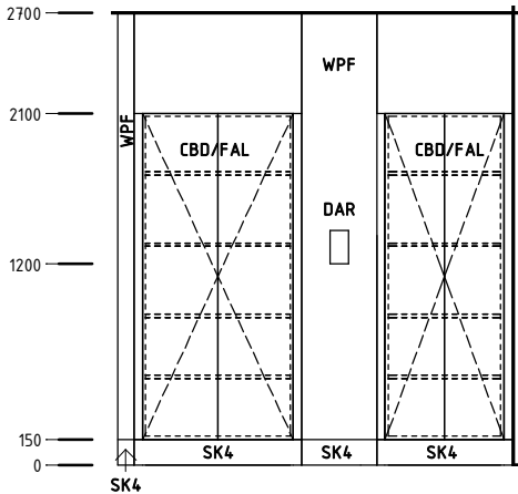
Elevation 2
