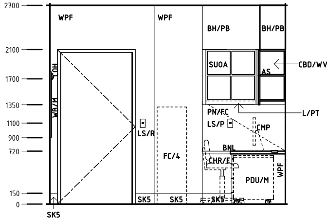
Elevation 3
