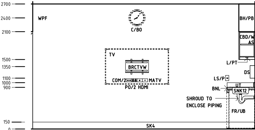
Elevation 2
