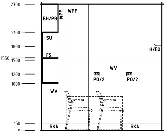
Elevation 3
