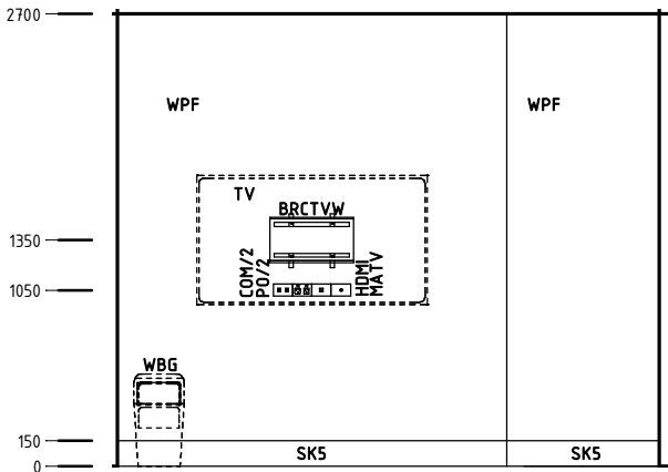
Elevation 4
