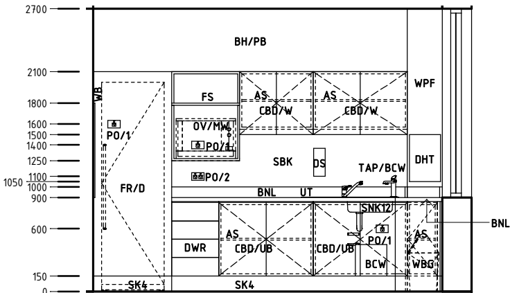
Elevation 2
