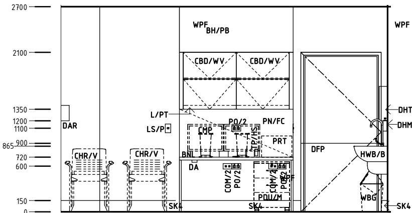
Elevation 1
