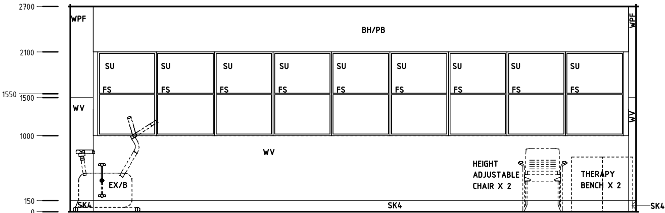
Elevation 2
