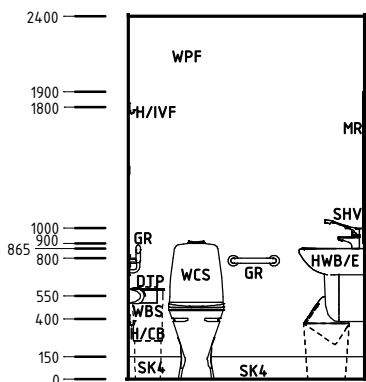
Elevation 3
