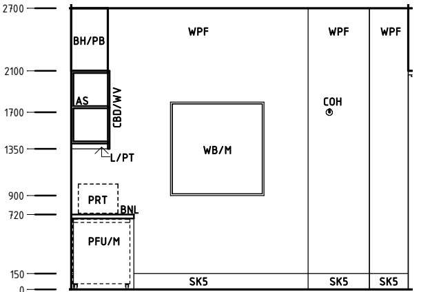
Elevation 4
