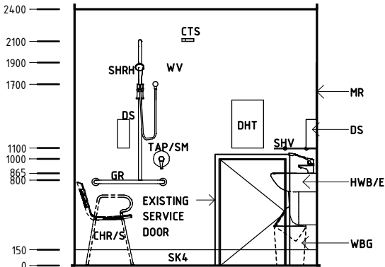
Elevation 3
