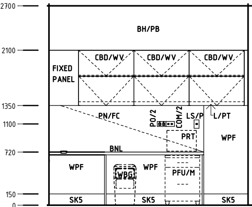
Elevation 3
