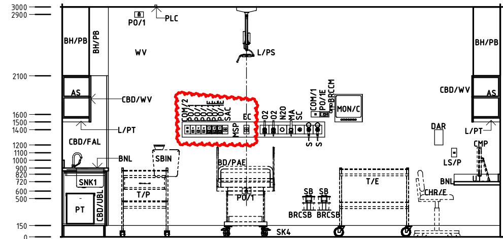
Elevation 3
