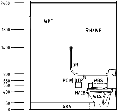
Elevation 4
